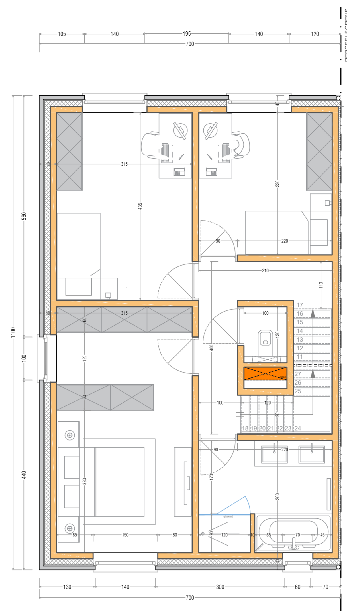
VERDIEPING 1
