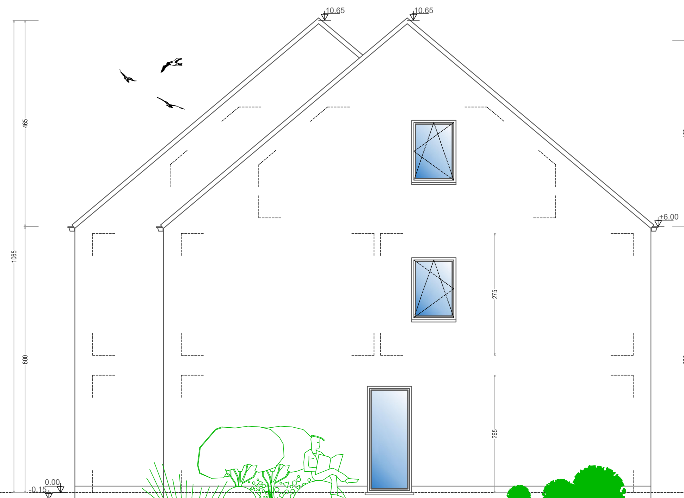
LINKER ZIJGEVEL
