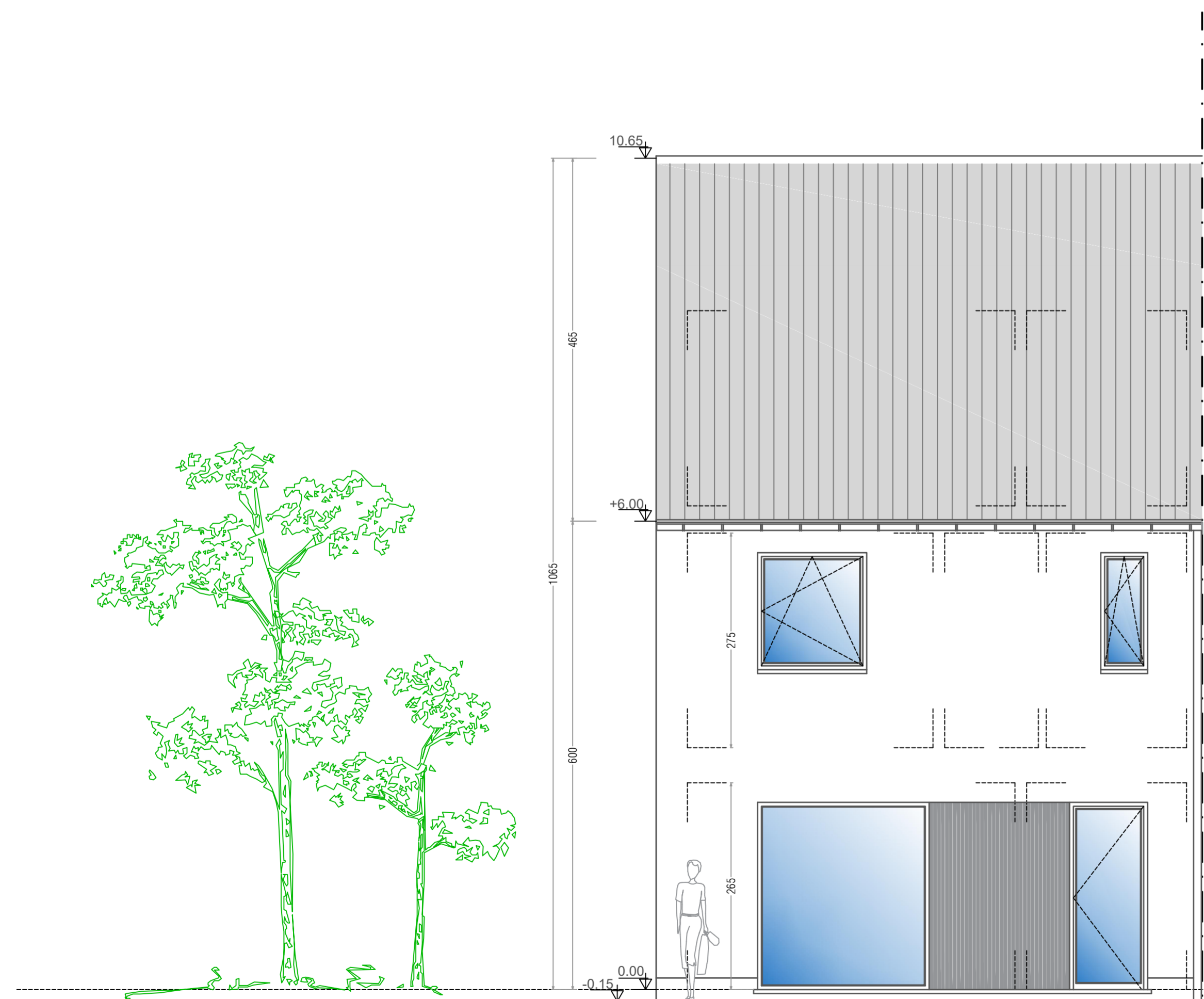
VOORGEVEL
