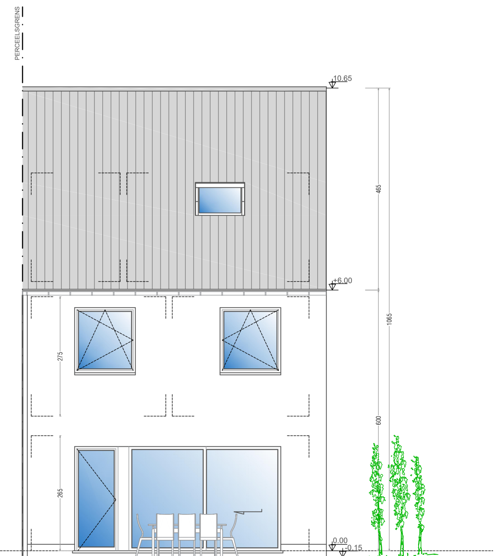
ACHTERGEVEL
