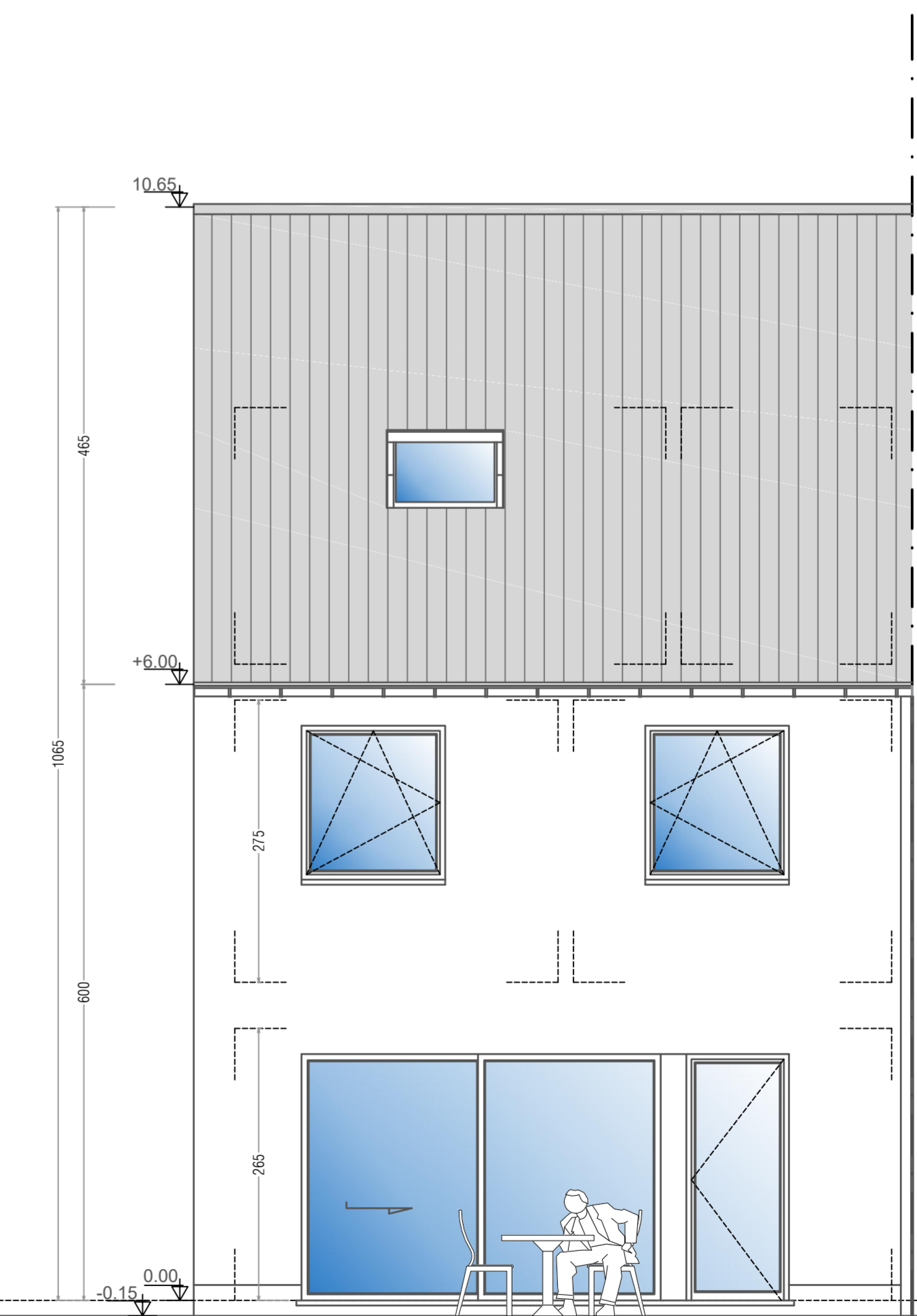
ACHTERGEVEL
