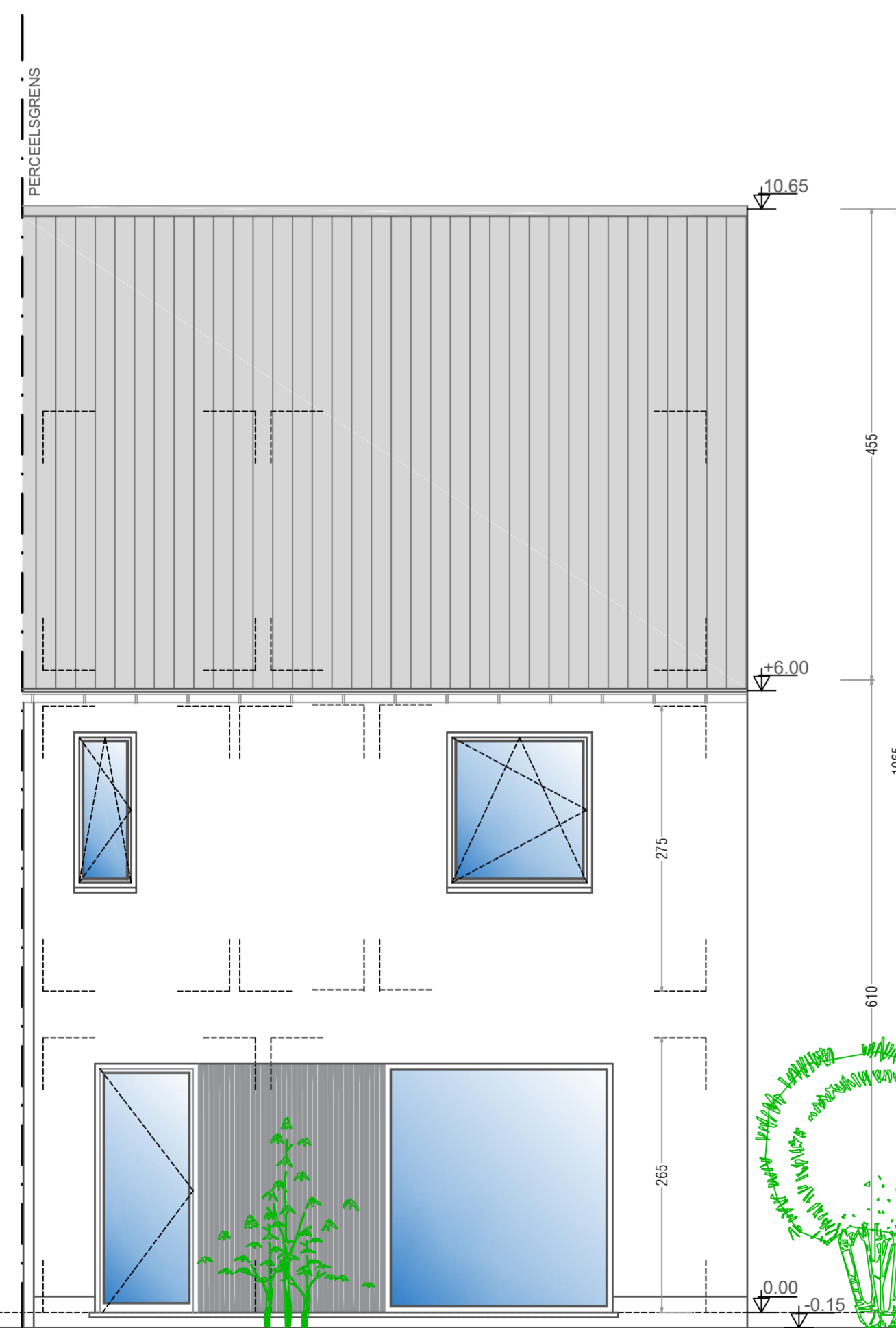
VOORGEVEL
