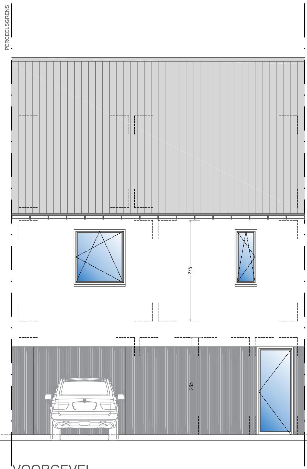
VOORGEVEL
