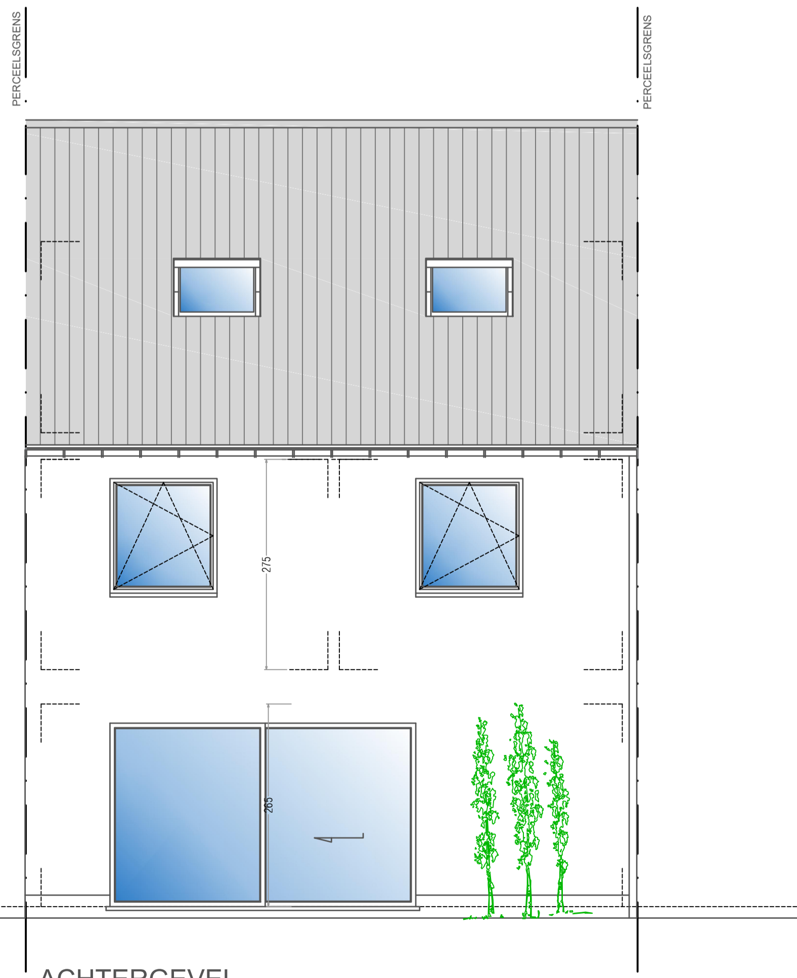
ACHTERGEVEL
