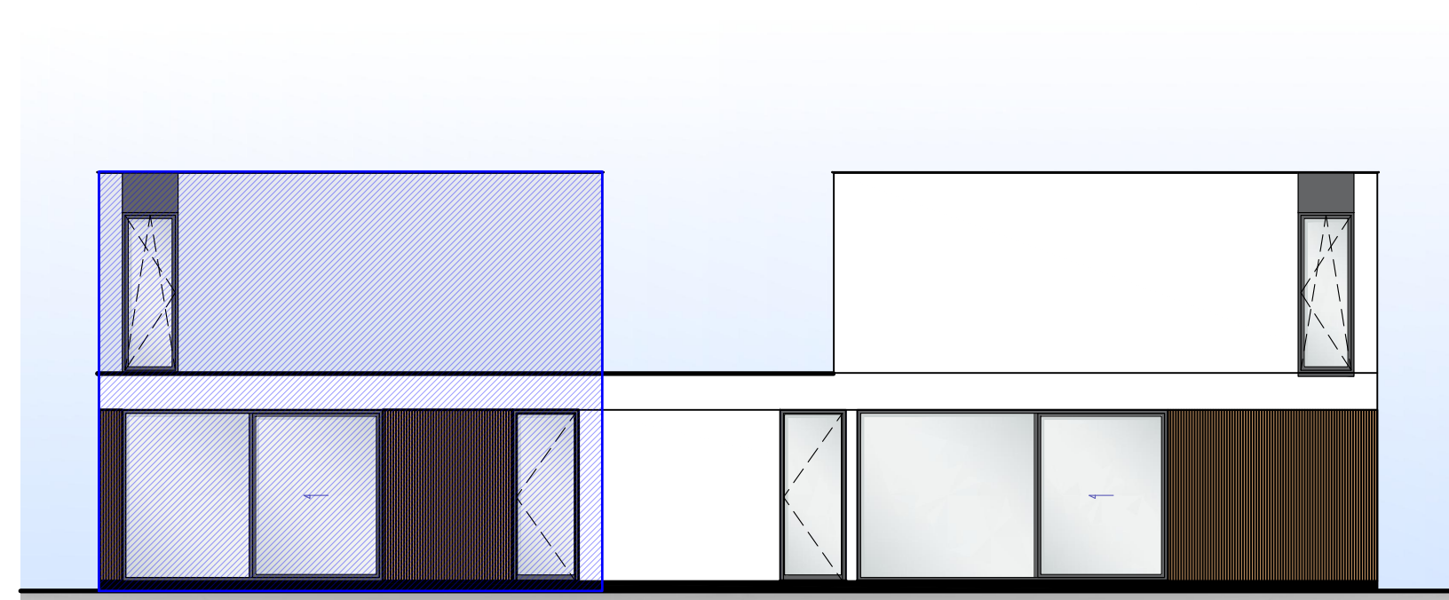
ACHTERGEVEL (WEST-NOORD-WEST) — ZICHT C
