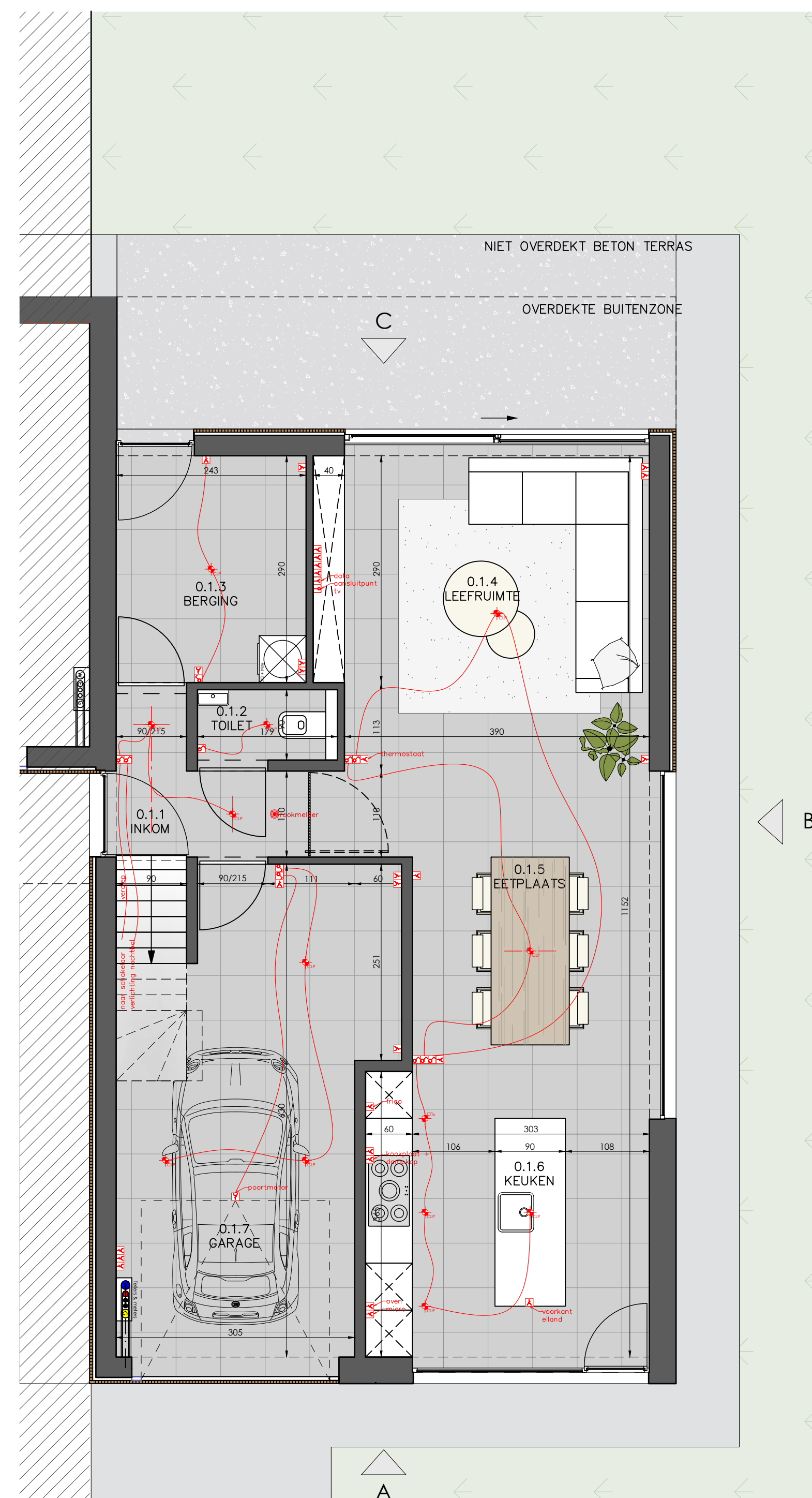
GELIJKVLOERS schaal 1/50
